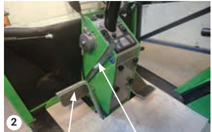
Brzdový pedál Parkovací brzda
